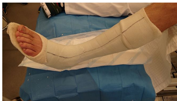
Linie zum Spalten des Gipses
